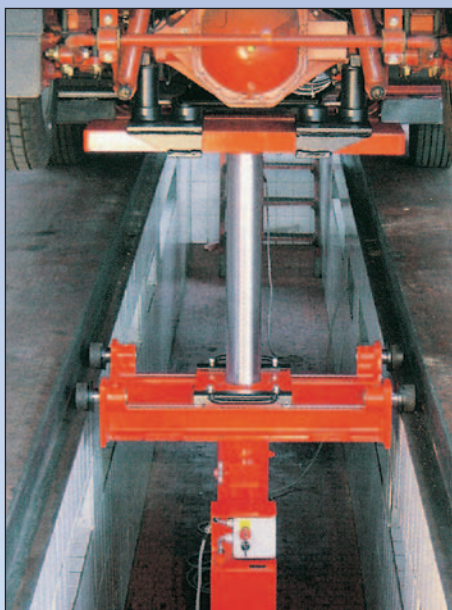
Einzelgrubenheber
